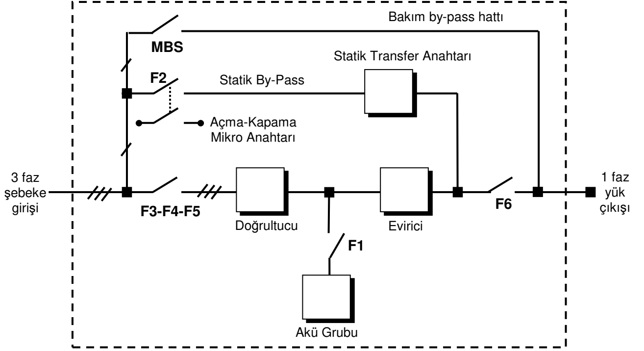
Şekil 1.1 Blok Diagram
