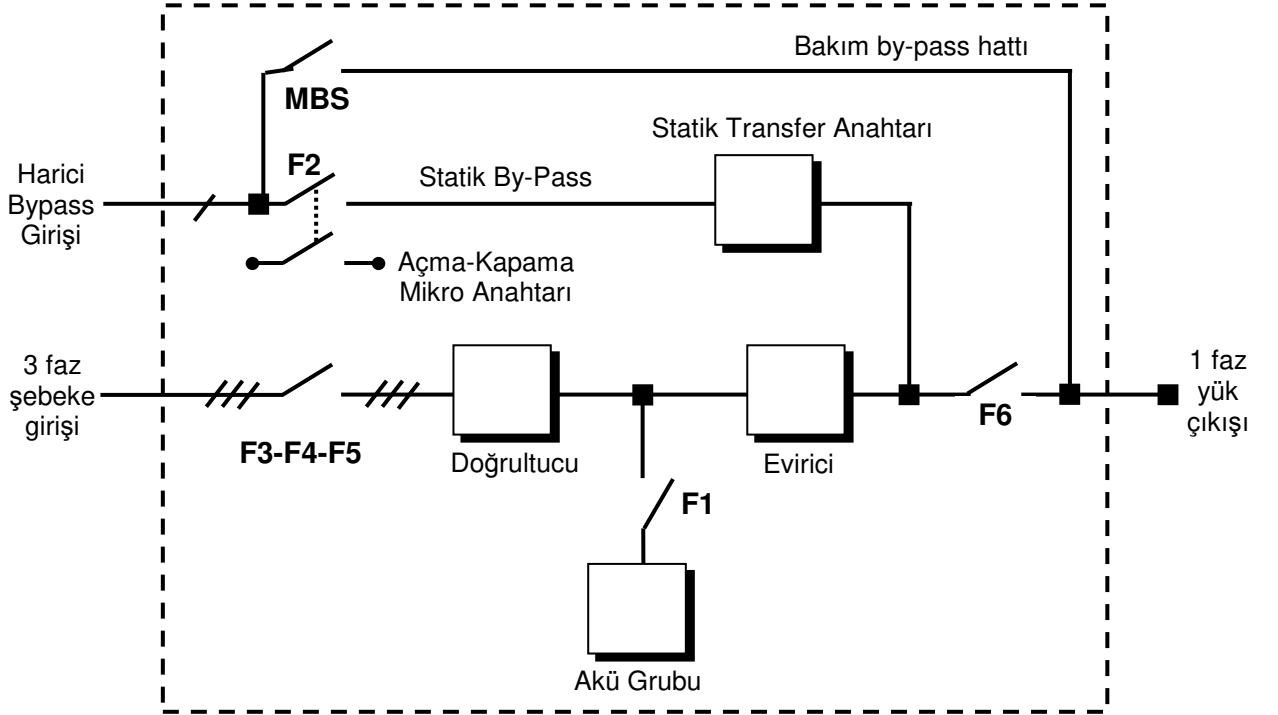
Şekil 1.2 Harici By-pass bağlantısı blok diagram
