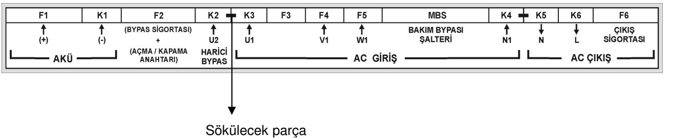
Şekil 5.2 Split (harici) By-Pass Kaynağı bağlantısı
