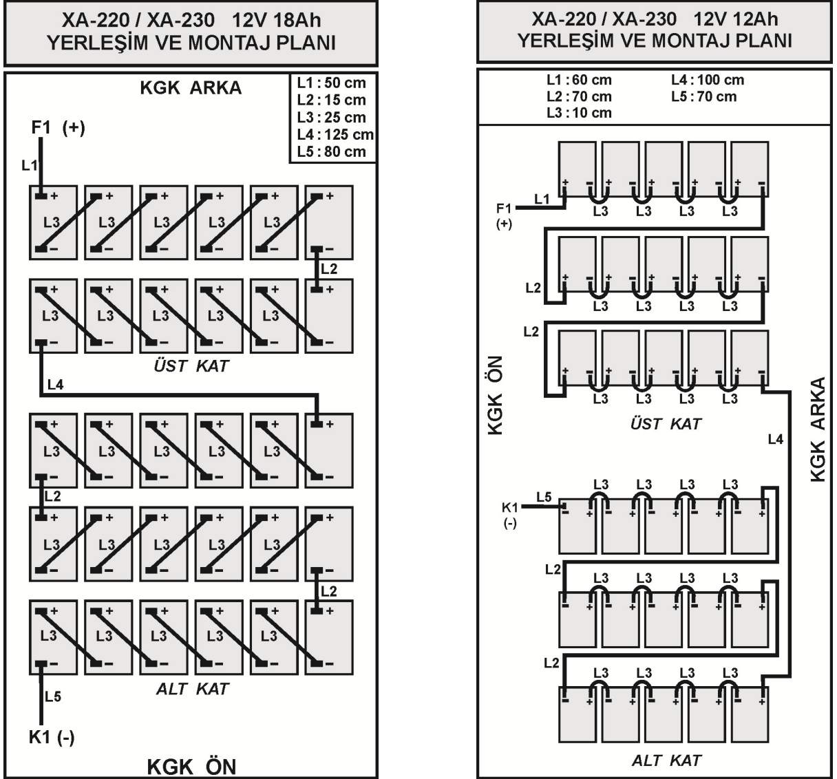
Şekil 5.3 KGK Akü Grubu Bağlantısı
