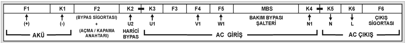
Şekil 5.1 Standart bağlantı
